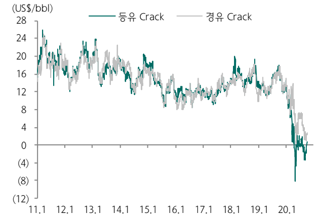
그림 96. 등/경유 Crack 추이
