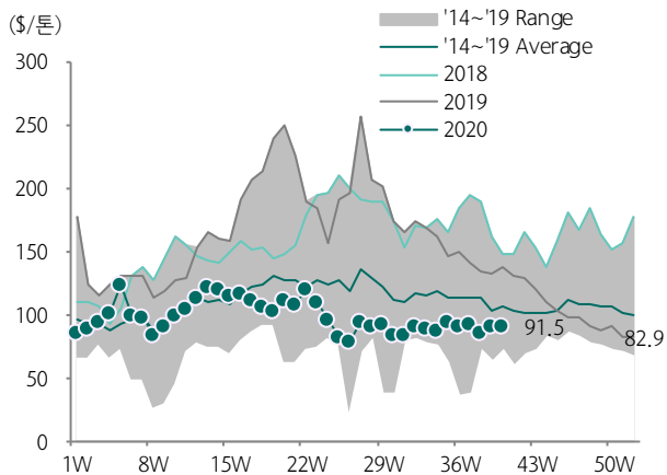
그림 37. PTA마진 추이(PX 차감 기준)
