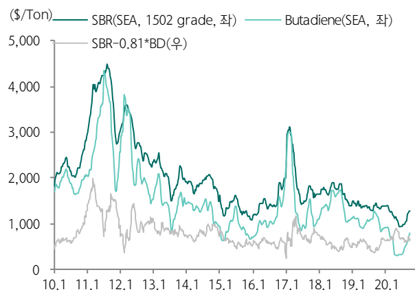
그림 87. SBR(Styrene Butadiene Rubber) 가격 및 Spread 추이
