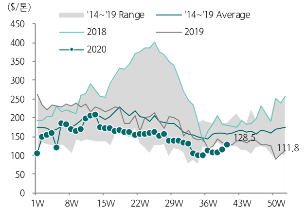
그림 36. PET마진 추이(MEG/PTA 차감 기준)
