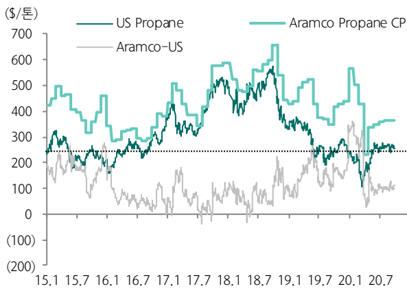
그림 19. 프로판 가격 추이. US 가격 WoW -4.14%
