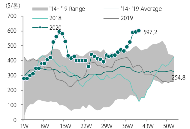
그림 46. PVC 마진 추이(납사 차감기준)
