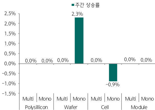
그림 9. 태양광 주요 체인별 제품가격 추이(PV Infolink 기준)
