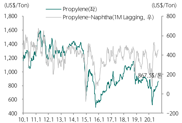
그림 71. 프로필렌 가격 및 Spread 추이
