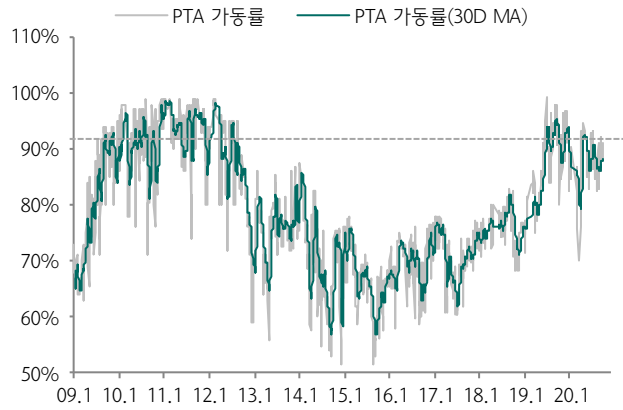
그림 28. 중국 PTA 가동률 91.3%
