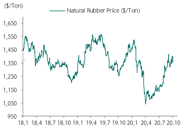
그림 38. 천연고무 가격 추이
