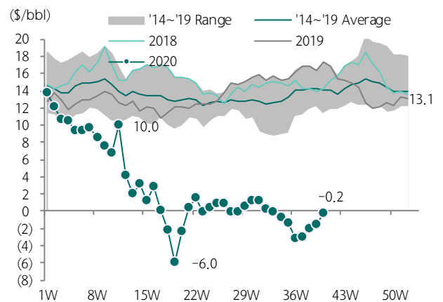
그림 50. 등유 마진 추이
