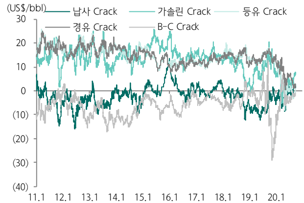
그림 94. 제품별 Crack 마진추이
